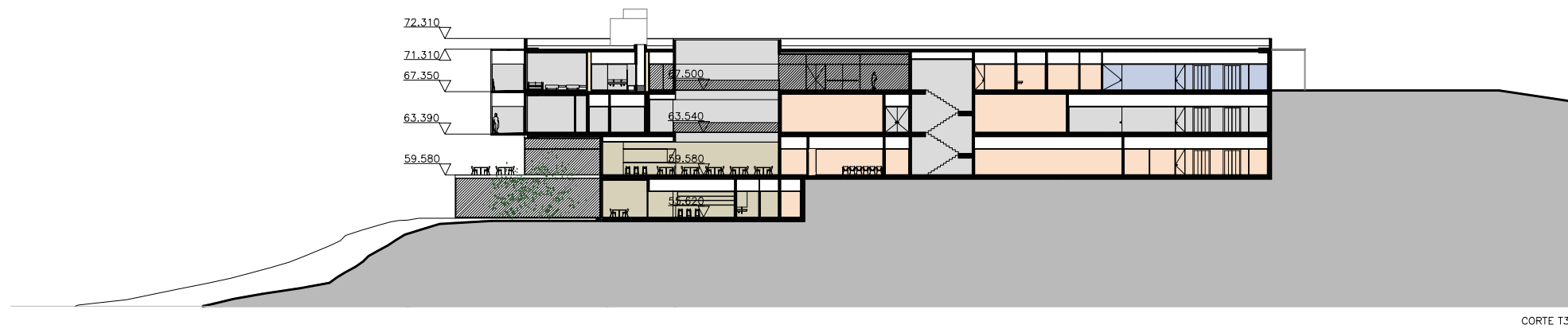
CORTE T3
