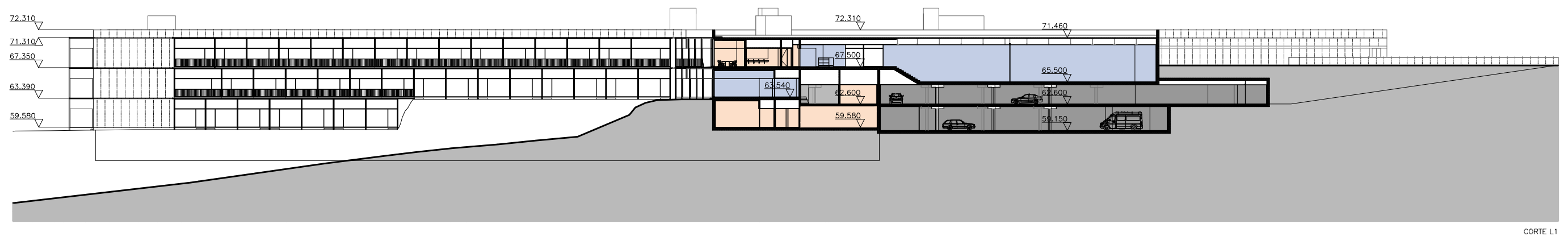
CORTE L1
