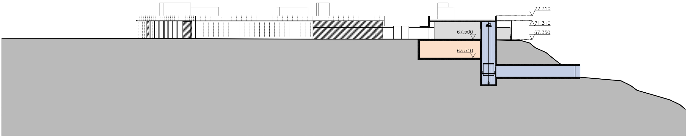
CORTE T1
