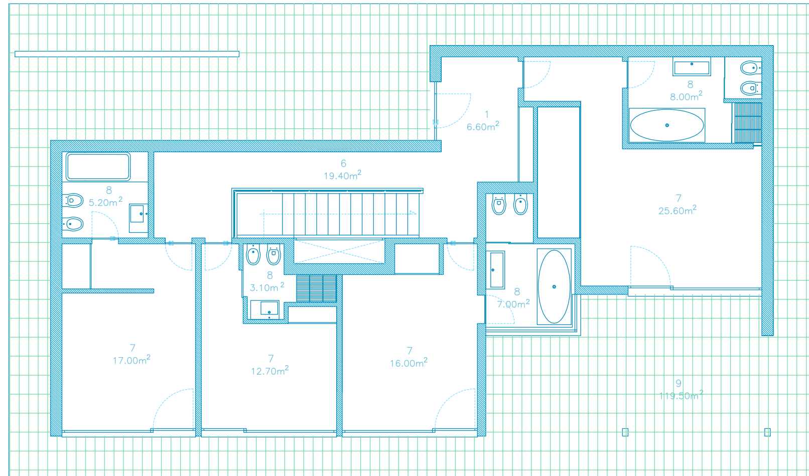
PLANTA PISO 0
