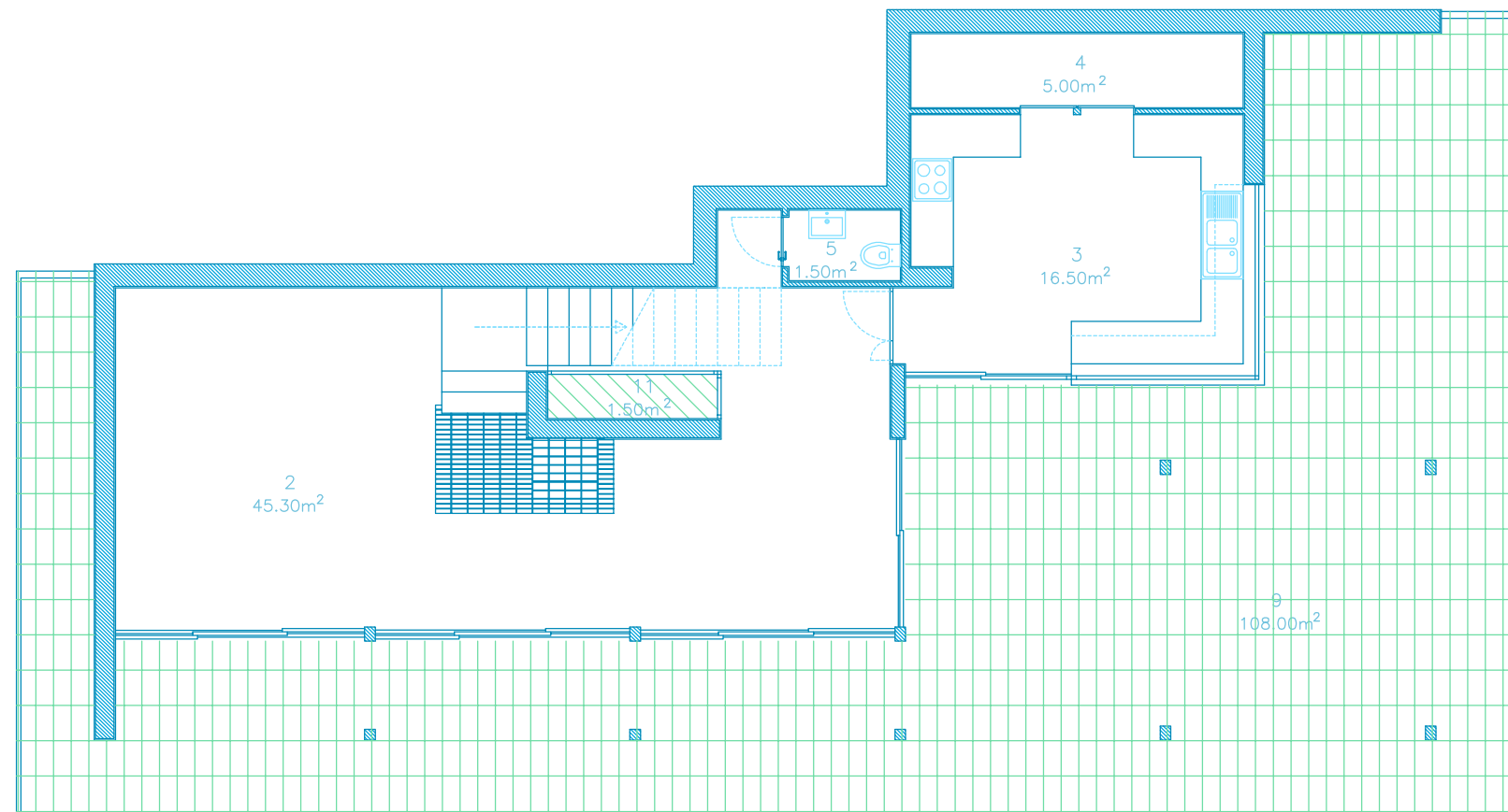
PLANTA PISO -1
