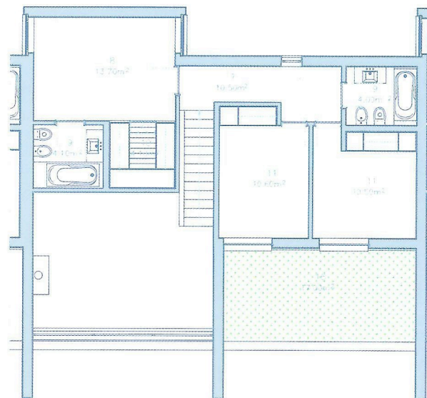
PLANTA PISO 1
