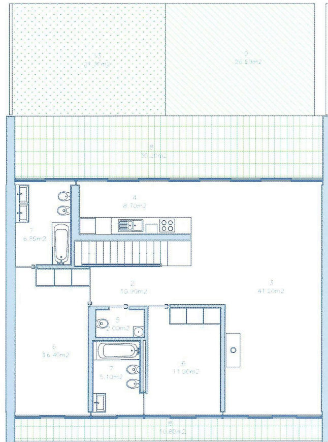
PLANTA PISO 0
