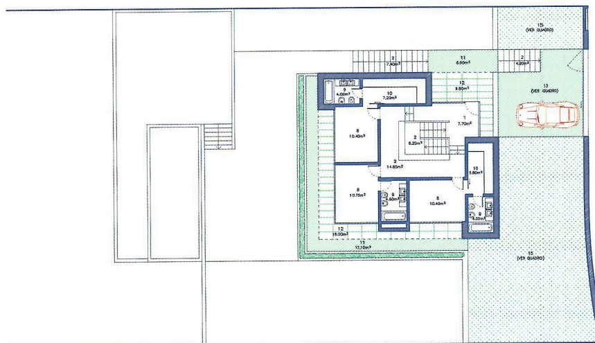
PLANO DEL PISO 1
