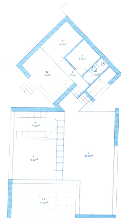
PLANTA DO PISO -1
